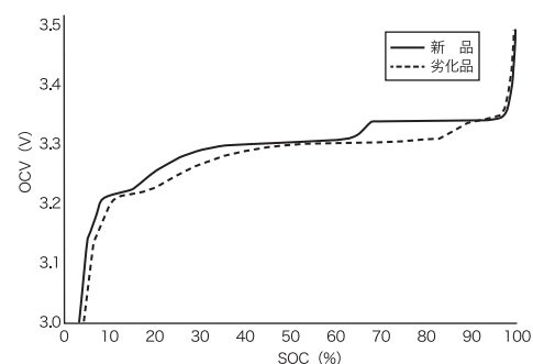
●図2 LFP電池のSOC-OCVプロファイル
