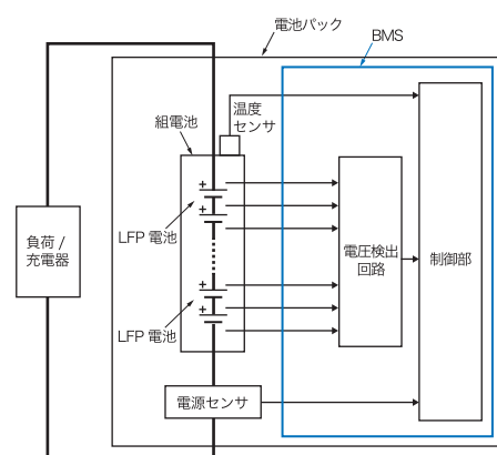
●図1 電池パックの概略
