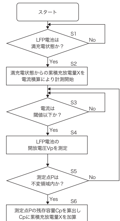
●図5 満充電容量推定のフローチャート
