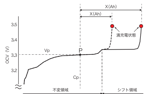
●図4 満充電状態からの累積充放電量
